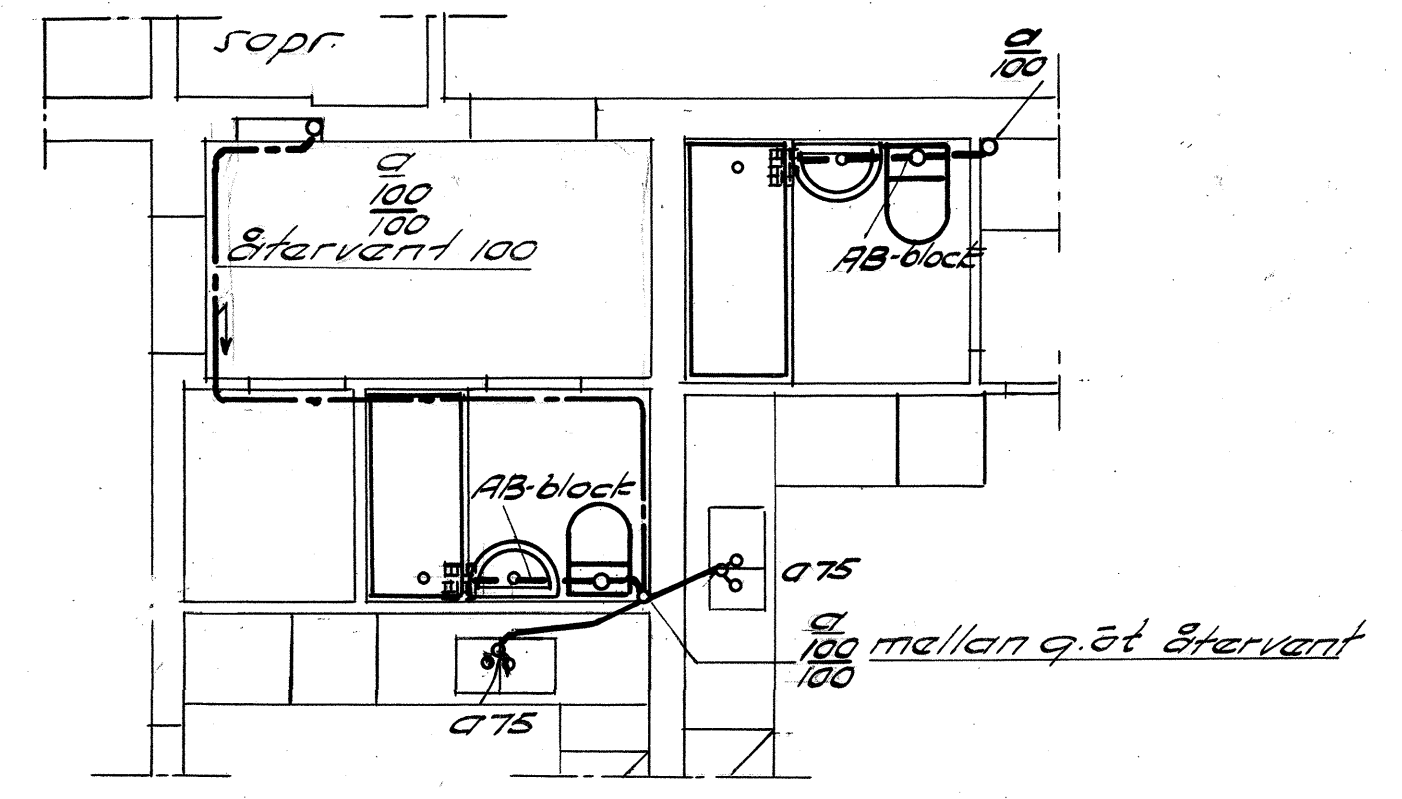
Detalj bad kök i trappor H. i. K.Ö.L.
